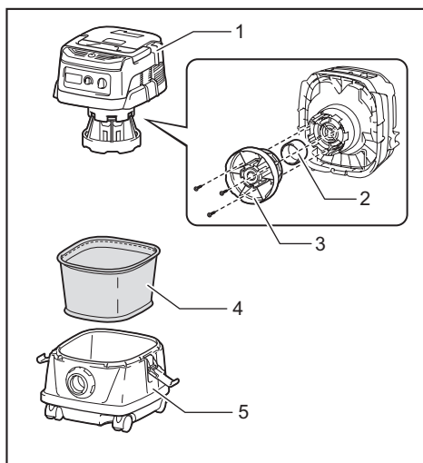
► 1. Cubierta del tanque 2. Flotador 3. Caja del flotador 4. Filtro de tela 5. Tanque
