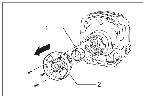
► 1. Float 2. Float cage
