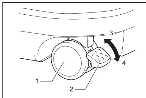
► 1. Rueda 2. Palanca del tope 3. Posición LIBERADA 4. Posición BLOQUEADA
