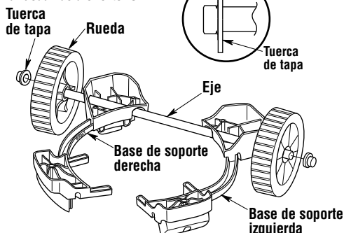
ENSAMBLAJE DE LAS BASES DE SOPORTE
