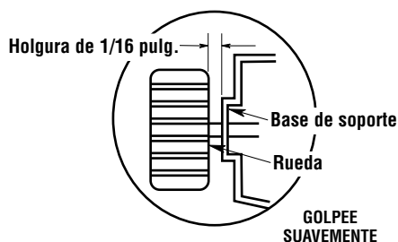
ENSAMBLAJE DE LAS BASES DE SOPORTE
